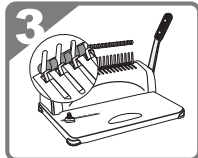
Apron seturut di balik piring sisir, Buka ke atas.
